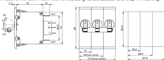
外形尺寸图
