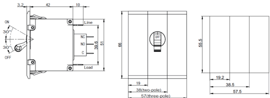
外形尺寸图
