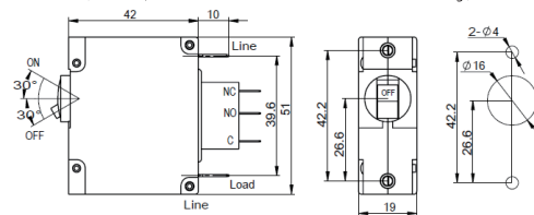
外形尺寸图
