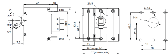
外形尺寸图
