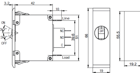
外形尺寸图
