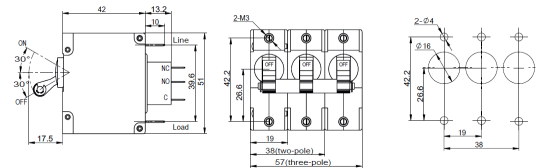
外形尺寸图 outline dimensions
