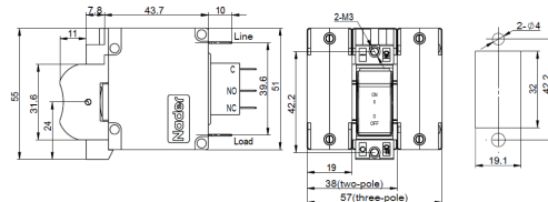
外形尺寸图
